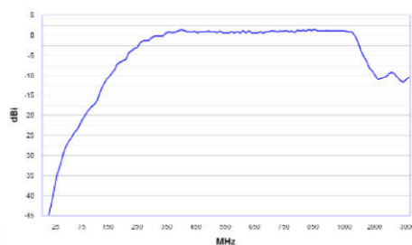
增益
