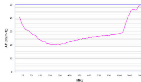
天线因子
