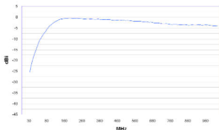
增益
