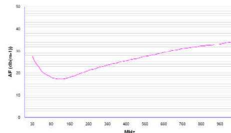
天线因子
