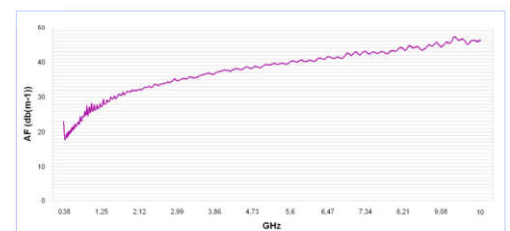
天线因子
