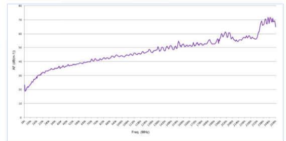
天线因子
