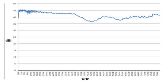
增益图
