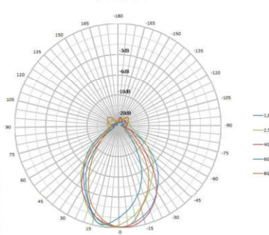
水平方向图
