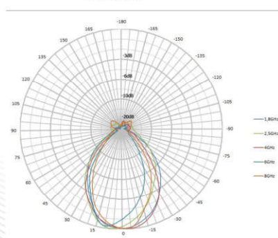
水平方向图
