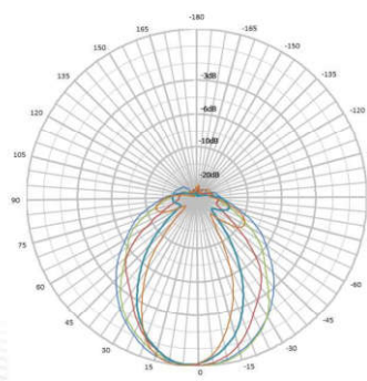
竖直方向图
