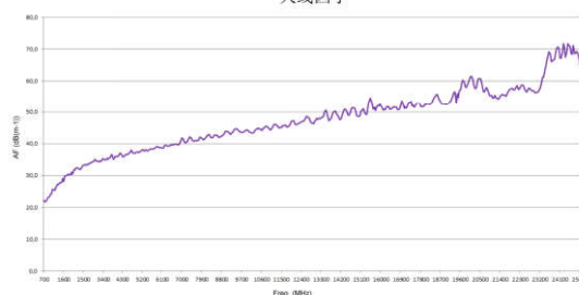
天线因子
