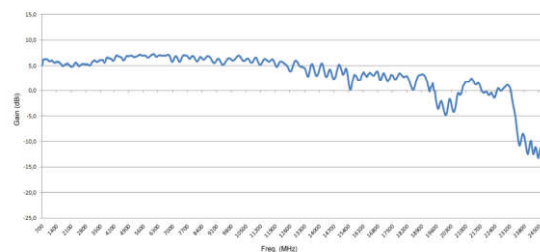
增益图
