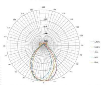
水平方向图
