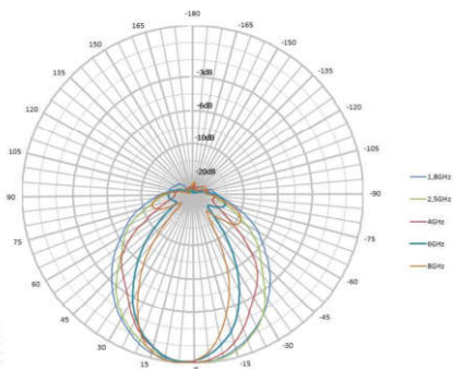
垂直方向图
