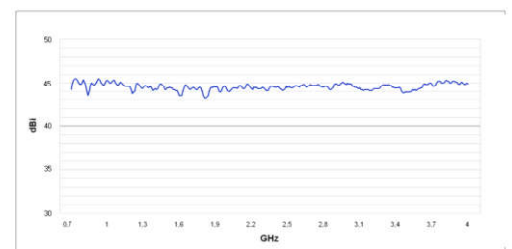
增益图
