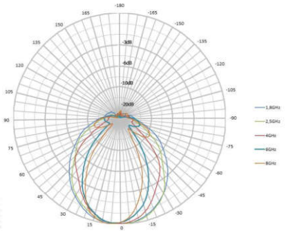
竖直方向图
