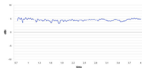
增益图
